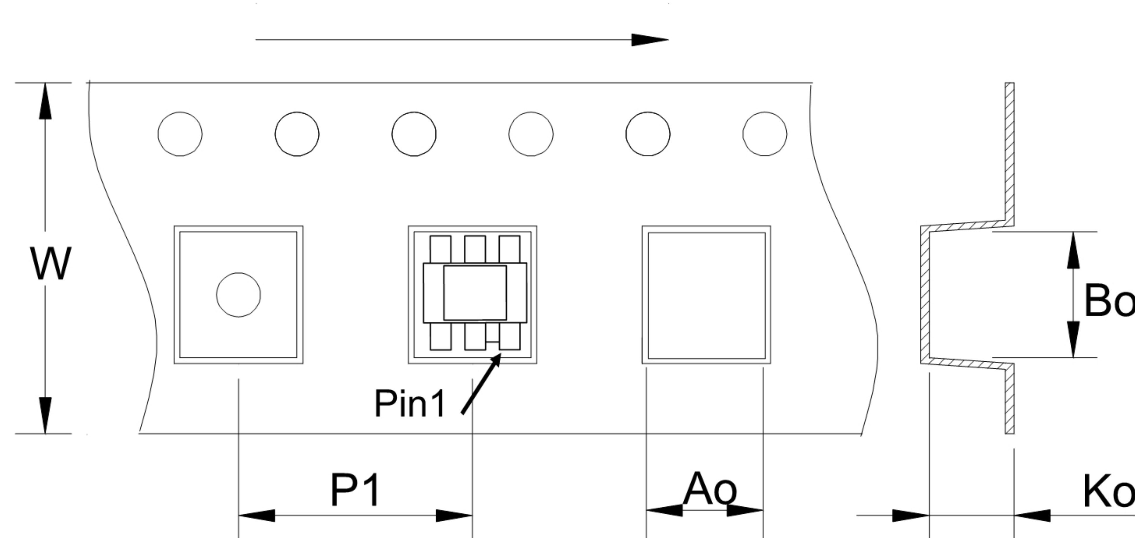
包装示意图
