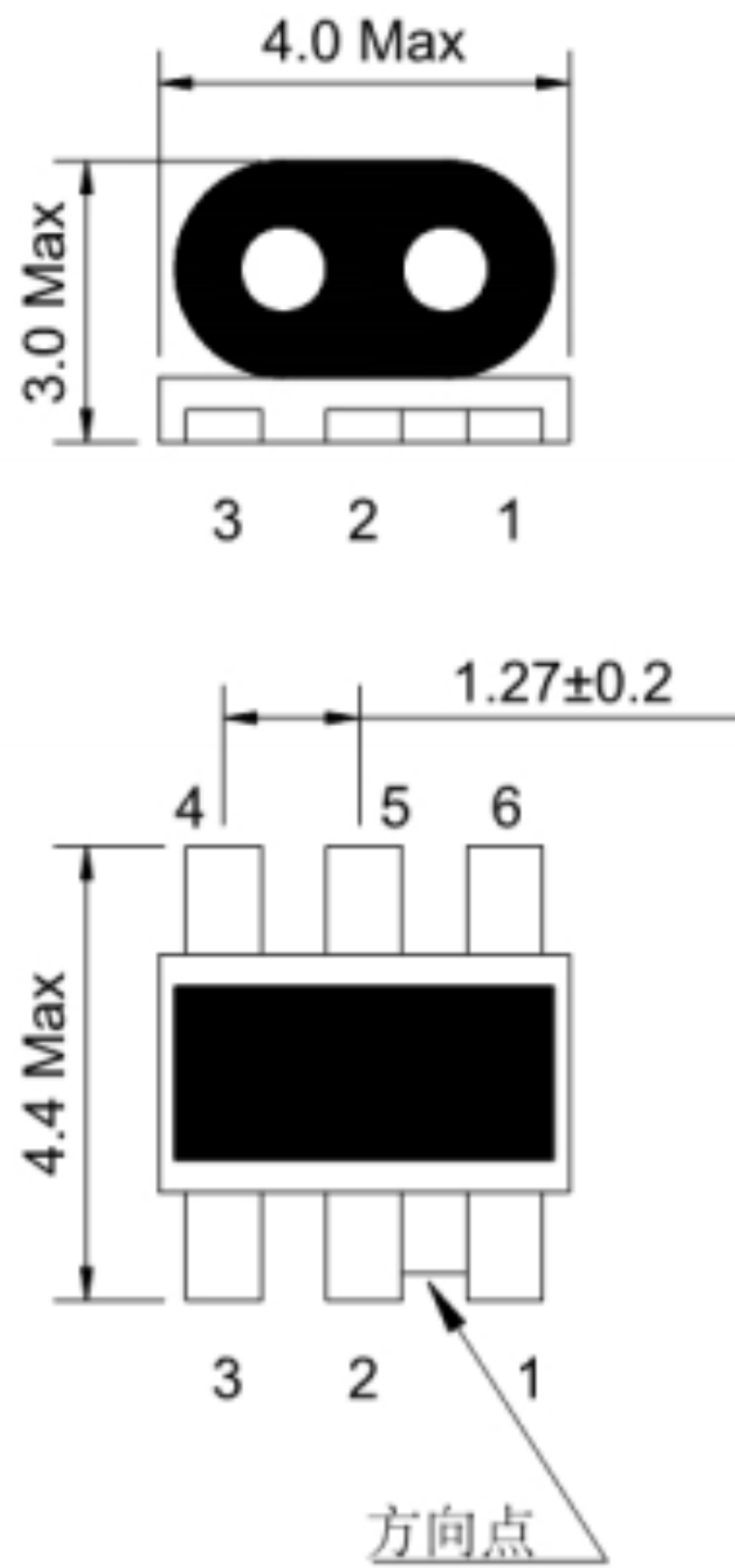
外形尺寸图(mm)
