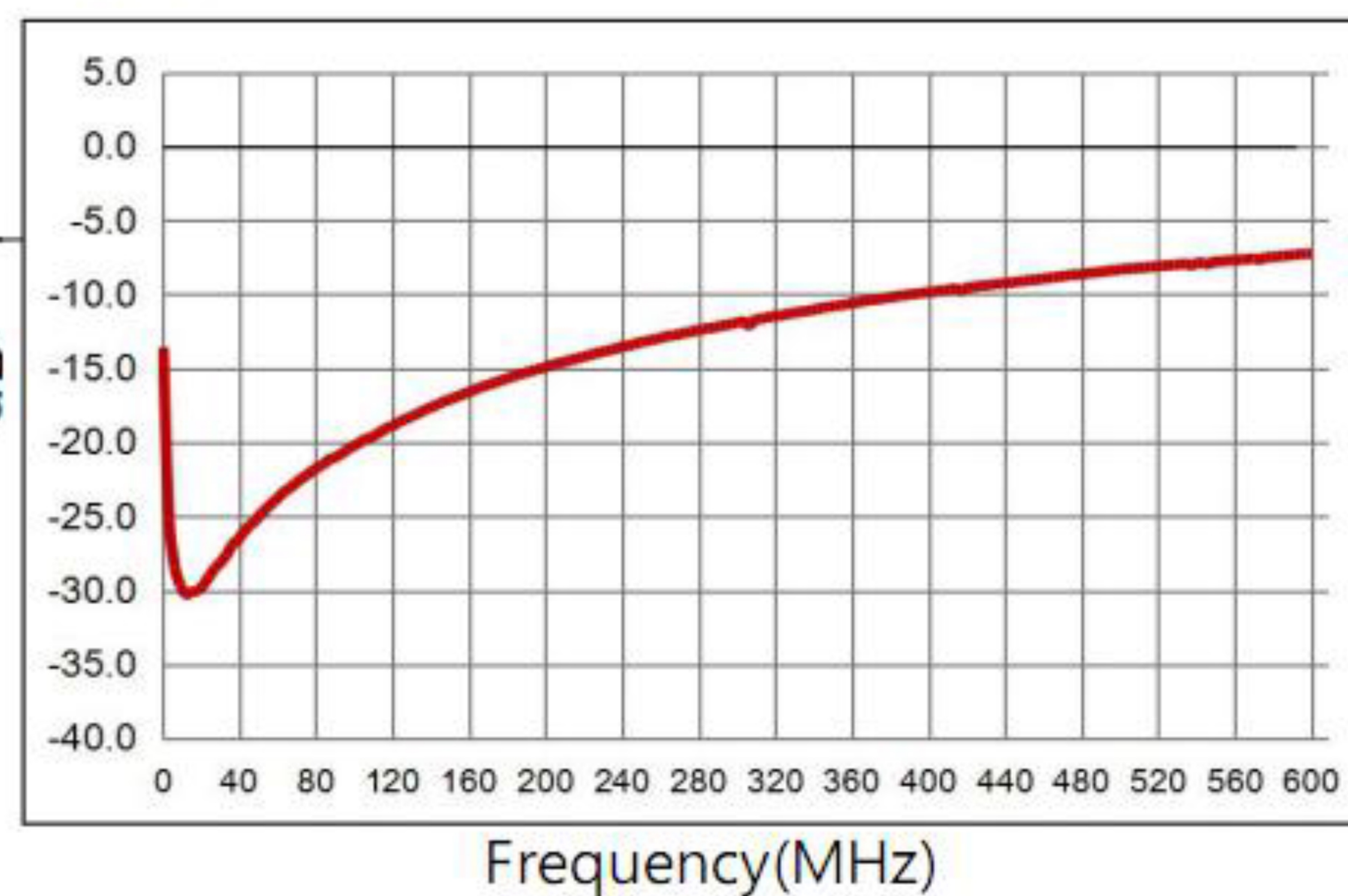
Sdd22
