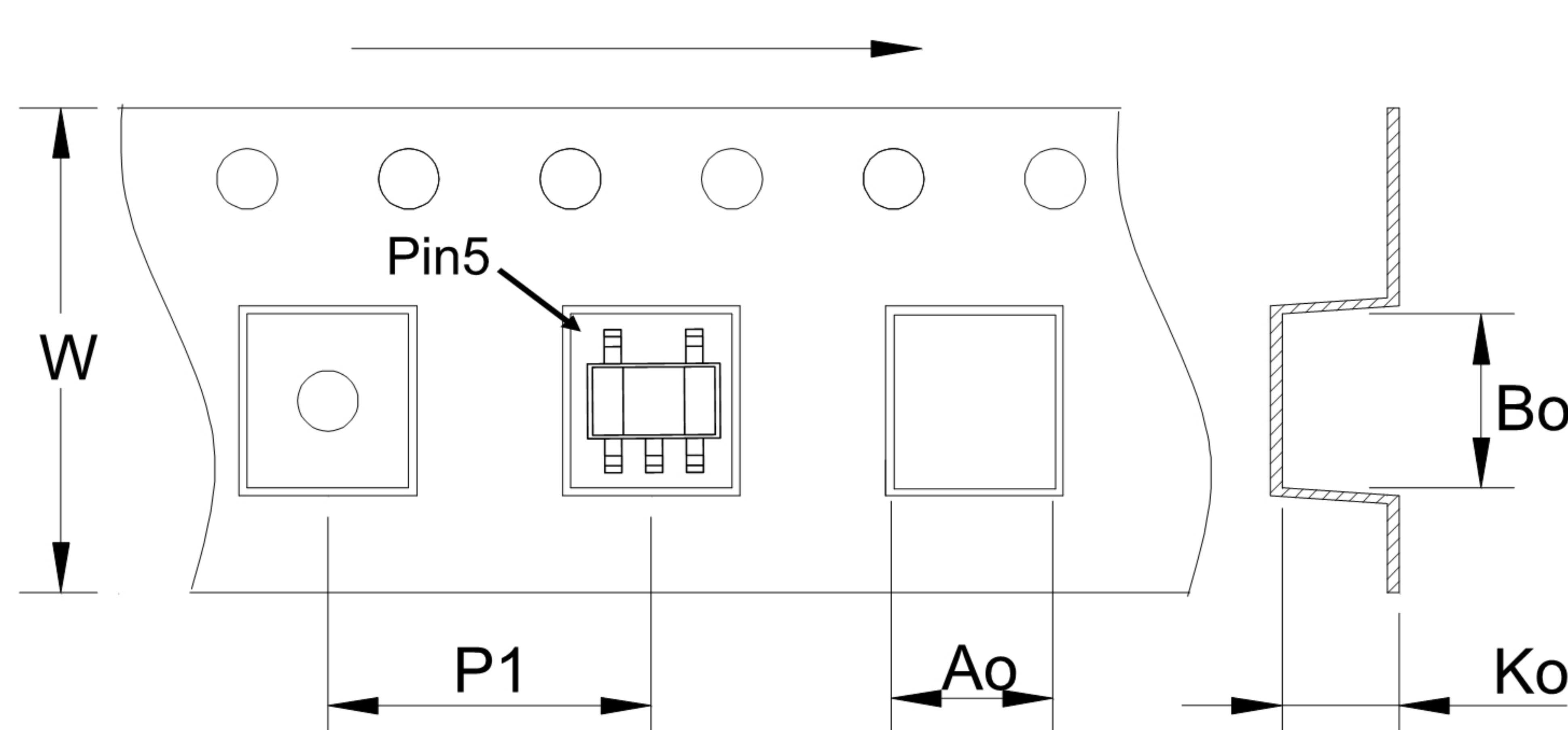
包装示意图
