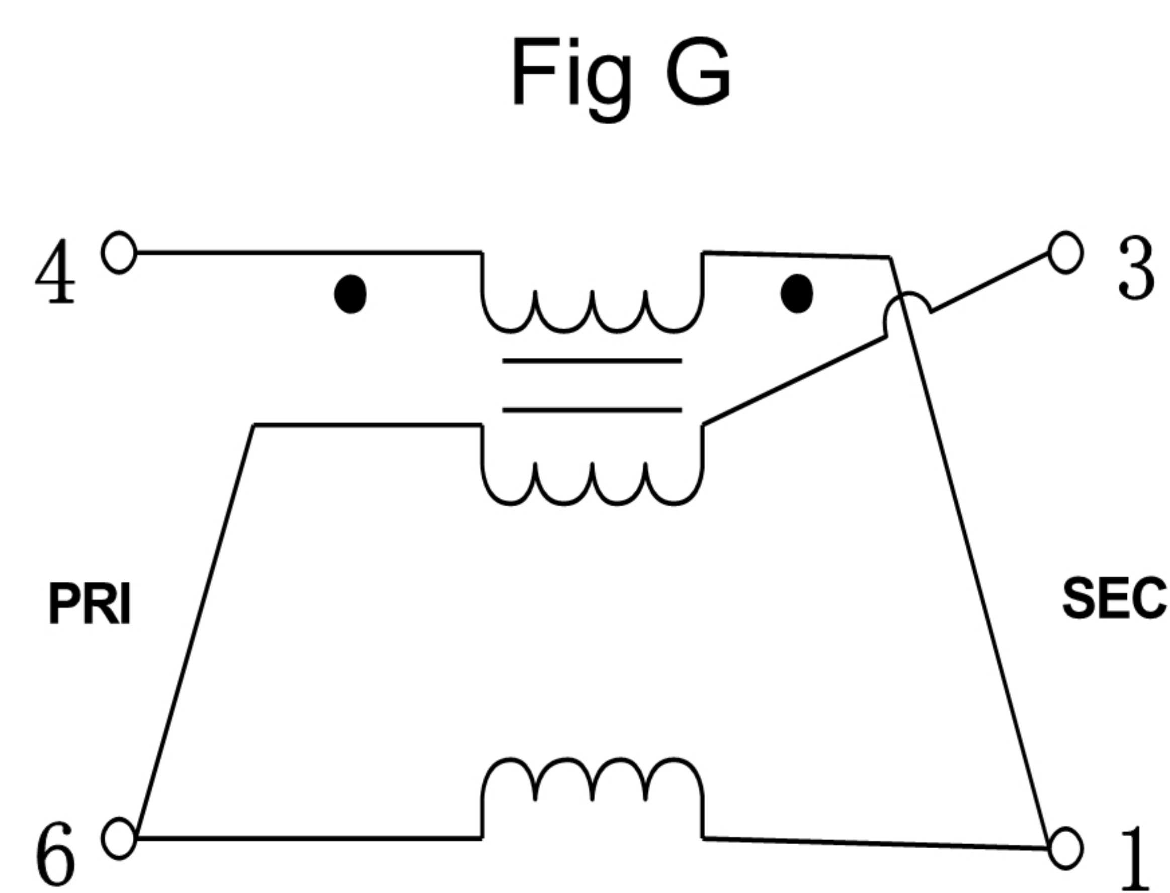
电气结构
