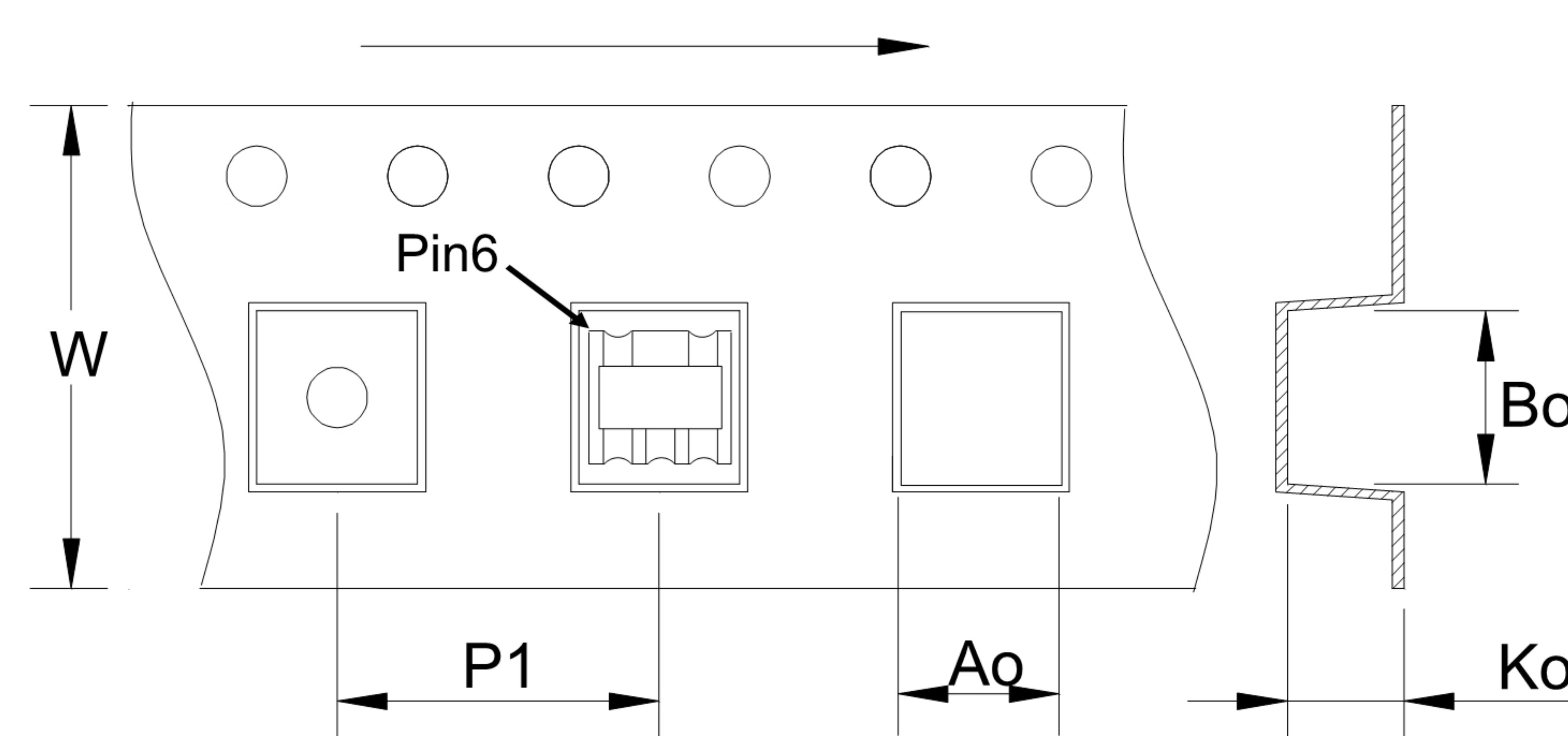
包装示意图
